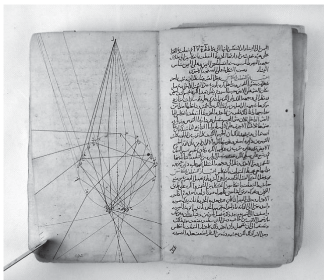
تصویر ۴. تصویری از نسخه‌ای از تنقیح المناظر ، توضیح و نمایش چگونگی شکست نور در کره شیشه‌ای
